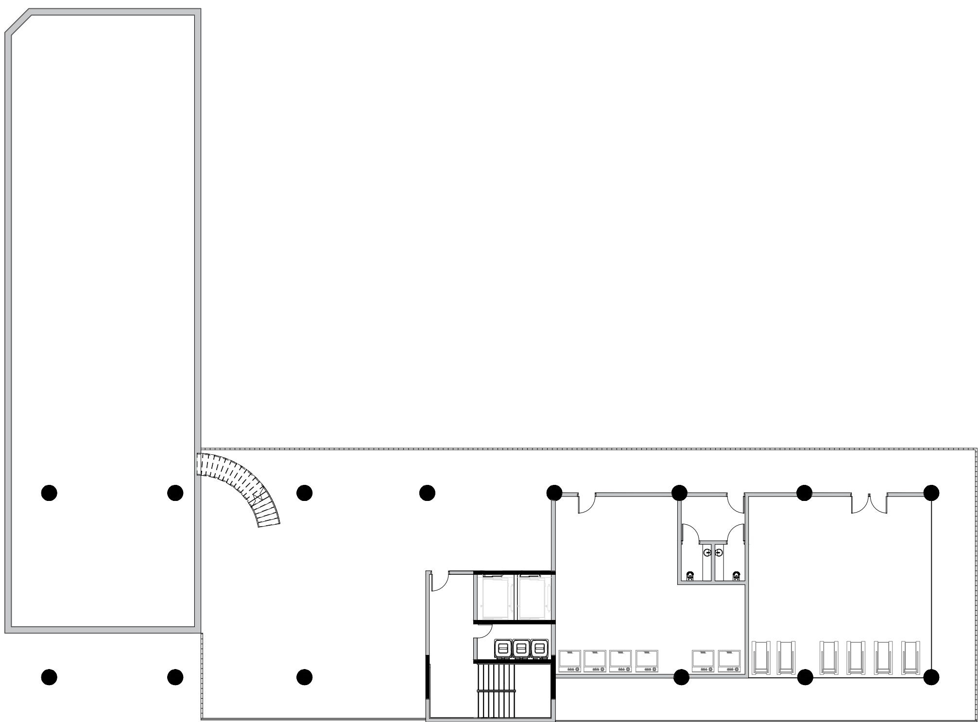
PLANTA TÉRREO + IMPLANTAÇÃO 1:200
