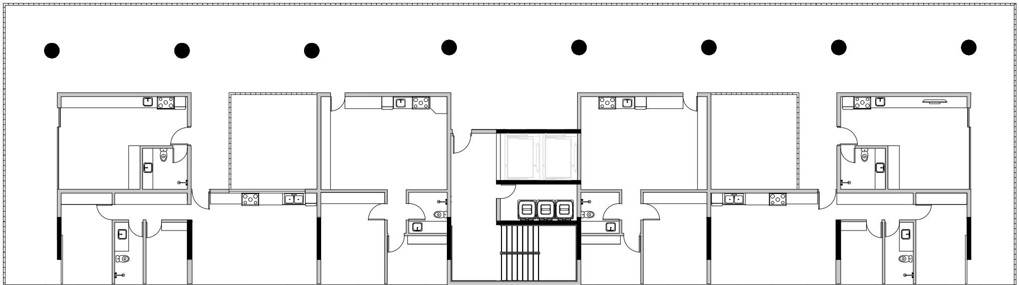
PLANTA PAVIMENTO TIPO 1:200
