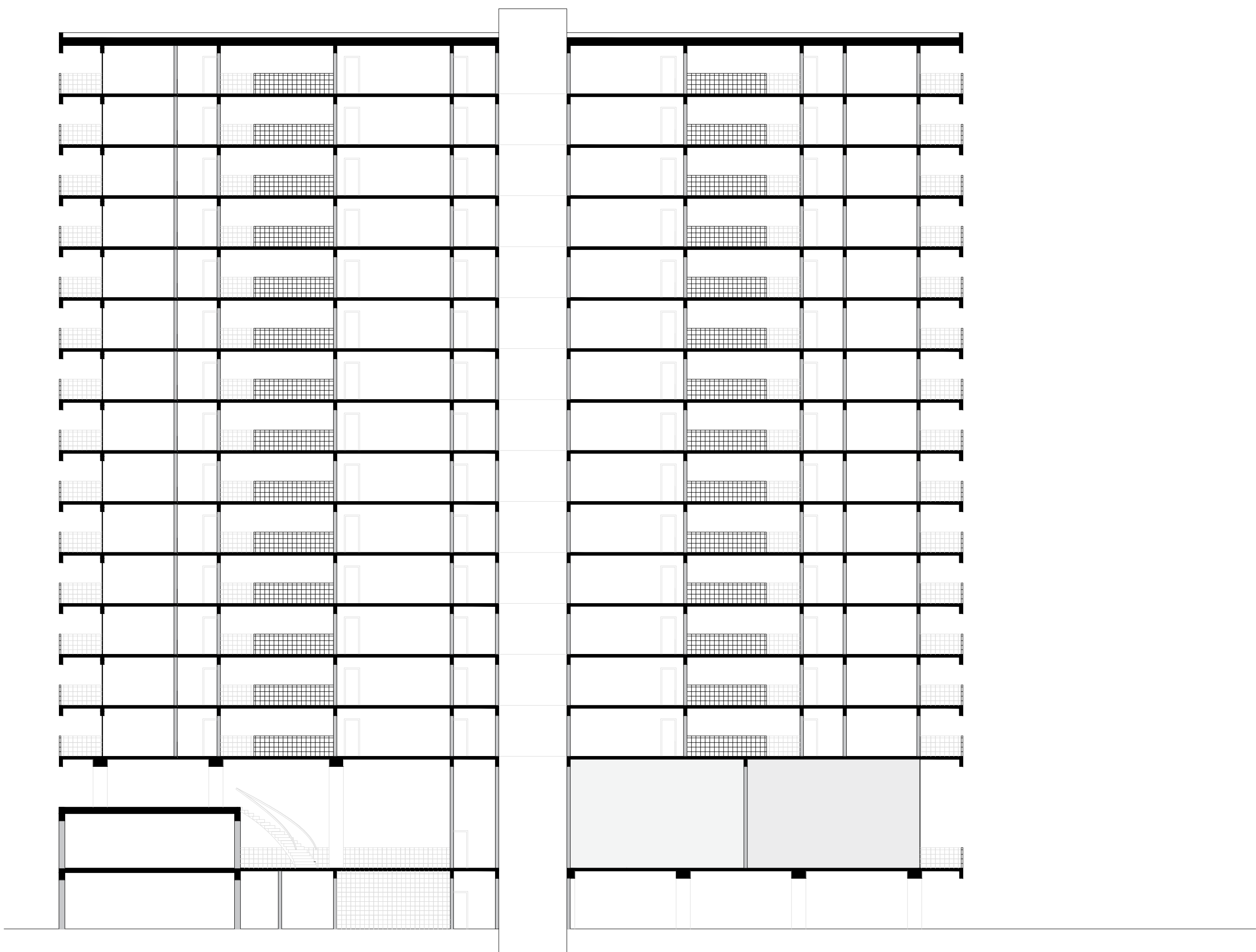
CORTE LONGITUDINAL 1:200
