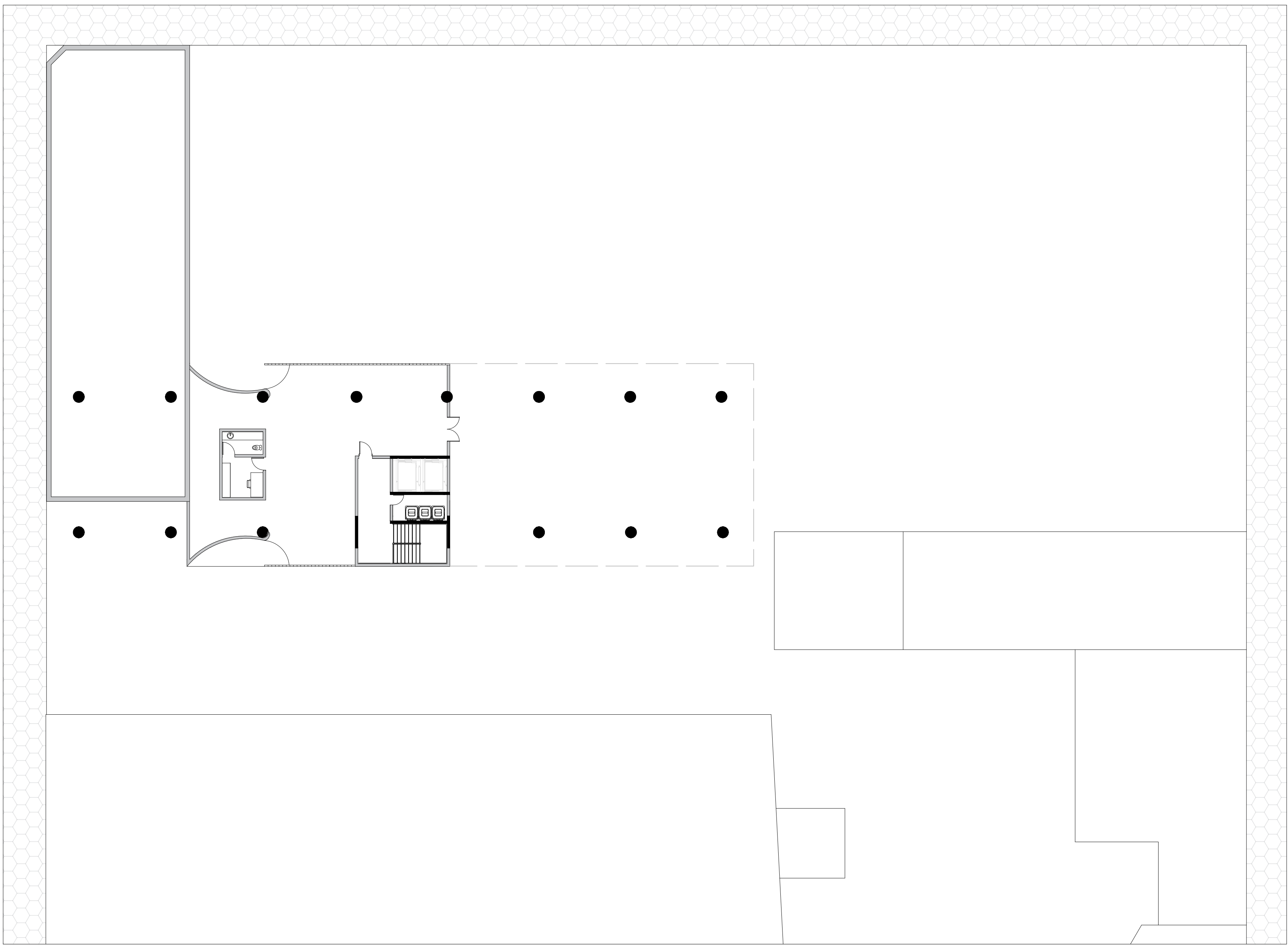
PLANTA TÉRREO + IMPLANTAÇÃO 1:200
